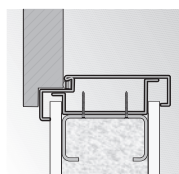
rohová zárubeň velká montáž do sádkartonové stěny
