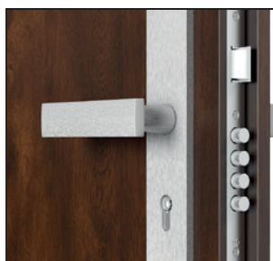
hlavní vícečepový zámek třídy 4 ENV
