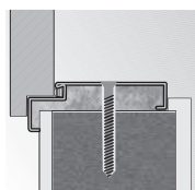
rohová zárubeň velká montáž pomocí hmoždinek
