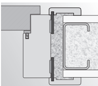
montáž do pěny do stěny ze sádrokartonové desky
