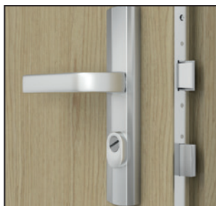
Čtyřbodový lištový zámek přizpůsobený pro dvě cylindrické vložky
