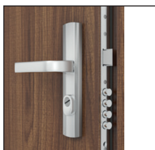
vícečepový lištový zámek přizpůsobený pro dvě cylindrické vložky
