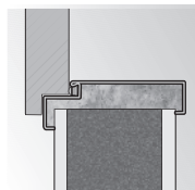
montáž bez dodatečných kotevících prvků
