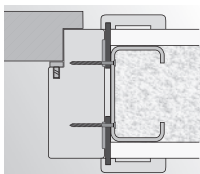
montáž na vruty do stěny ze sádrokartonové desky
