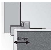
rohová zárubeň malá
