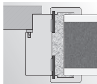
montáž do pěny do zděné stěny
