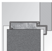
AGAT Montáž bez dodatečných kotvicích prvků
