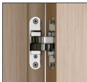
skrytý závěs 3D
