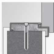
OPAL Montáž pomocí hmoždinek
